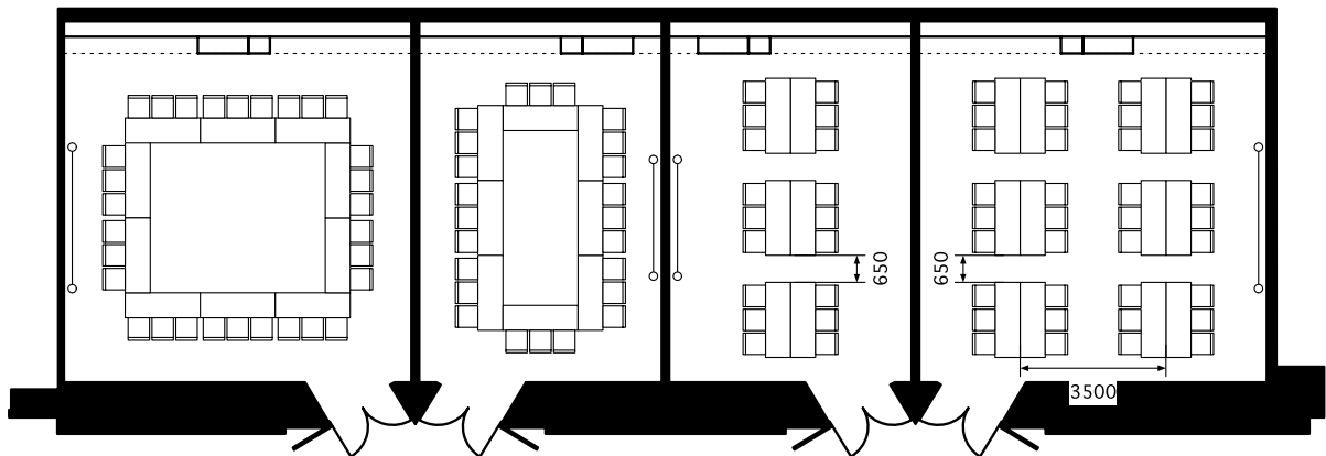
601・604会議室 スクリーン3600×2700 602・603会議室 スクリーン3000×2700
