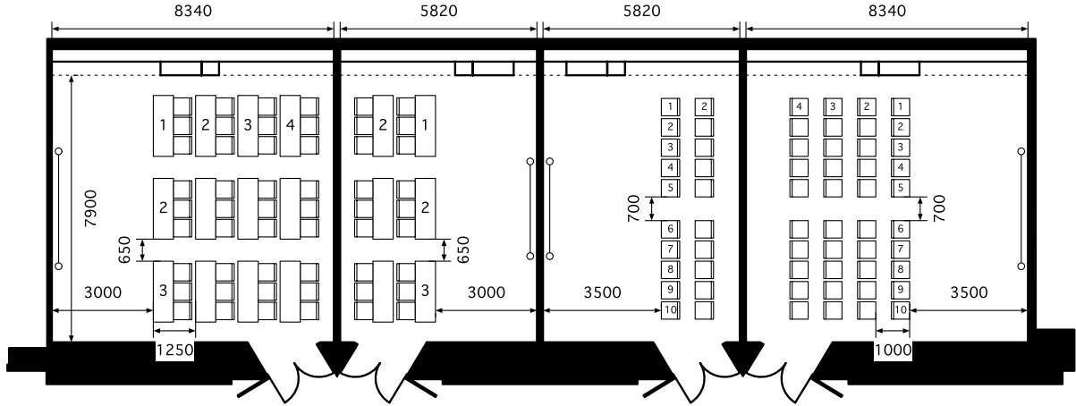
601・604会議室 スクリーン3600×2700 602・603会議室 スクリーン3000×2700
