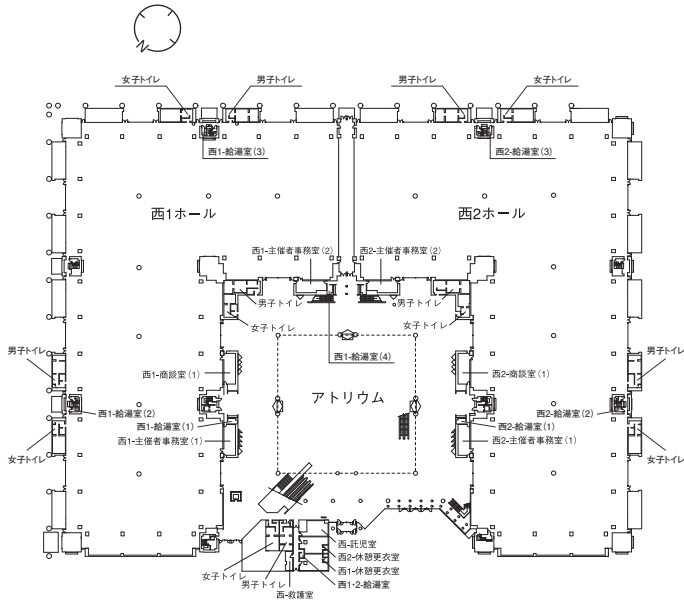
1F全体図
