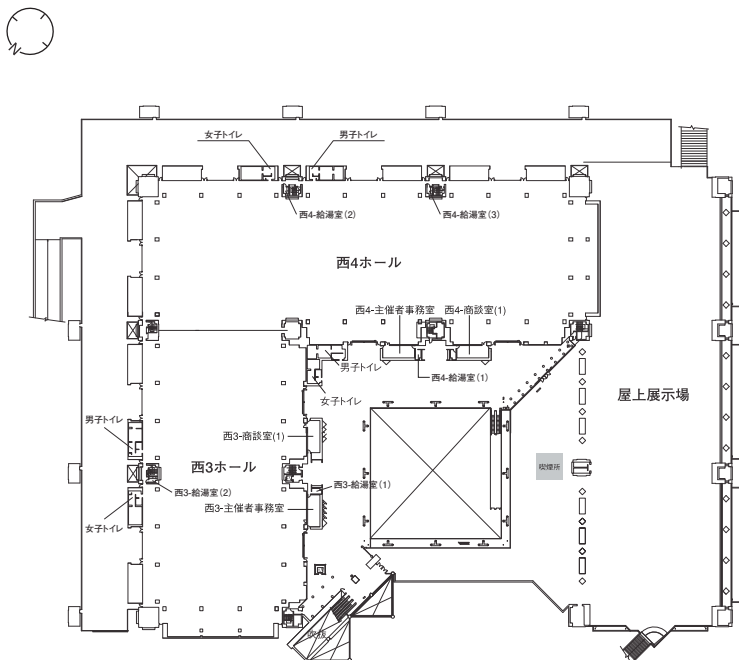
4F全体図
