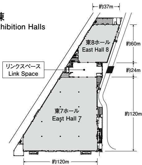
平面図 Floor Plan
